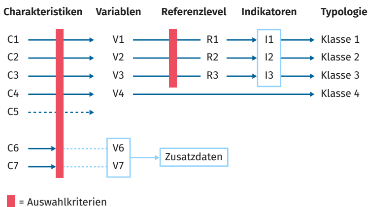
Abbildung 3: Schematischer Ablauf von Charakteristiken der Ökosysteme. Beginnend mit der Auswahl von Variablen über das potenzielle Hinzufügen von Referenzleveln bis hin zur Einordnung in die Zustandstypologie, verändert nach Keith H. et al. 2020 5
